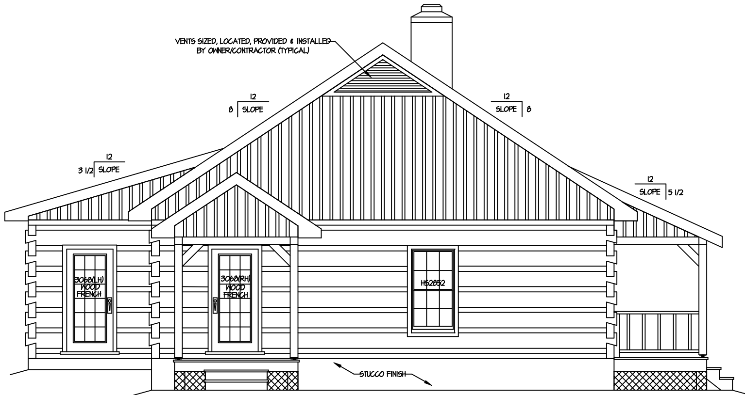
PLAN LEFT
