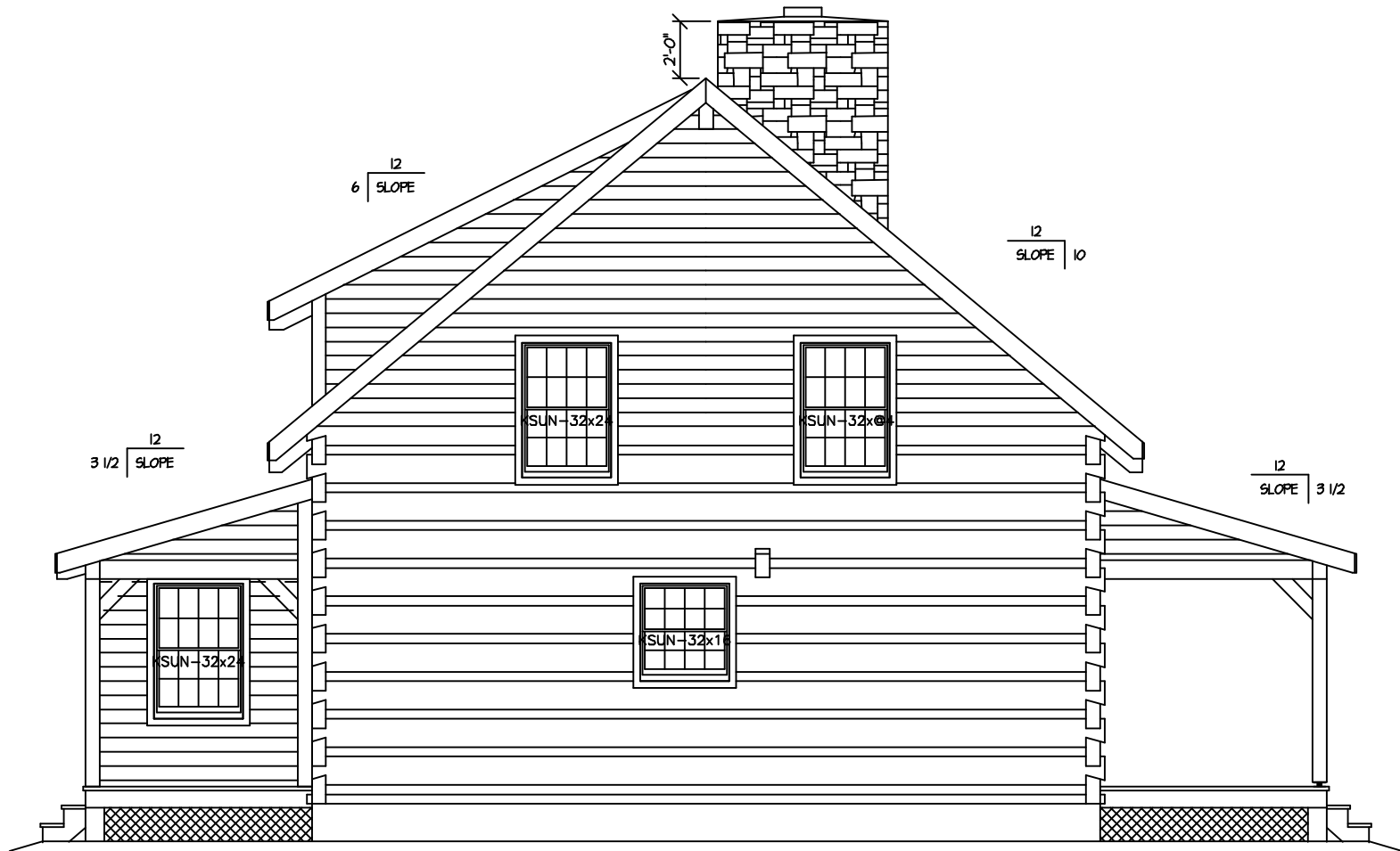
PLAN LEFT
