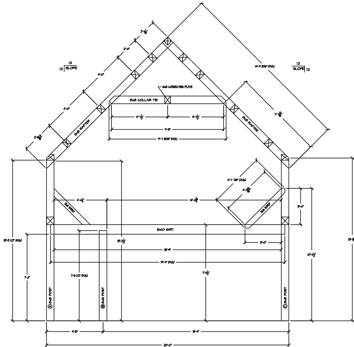
BENT #3
