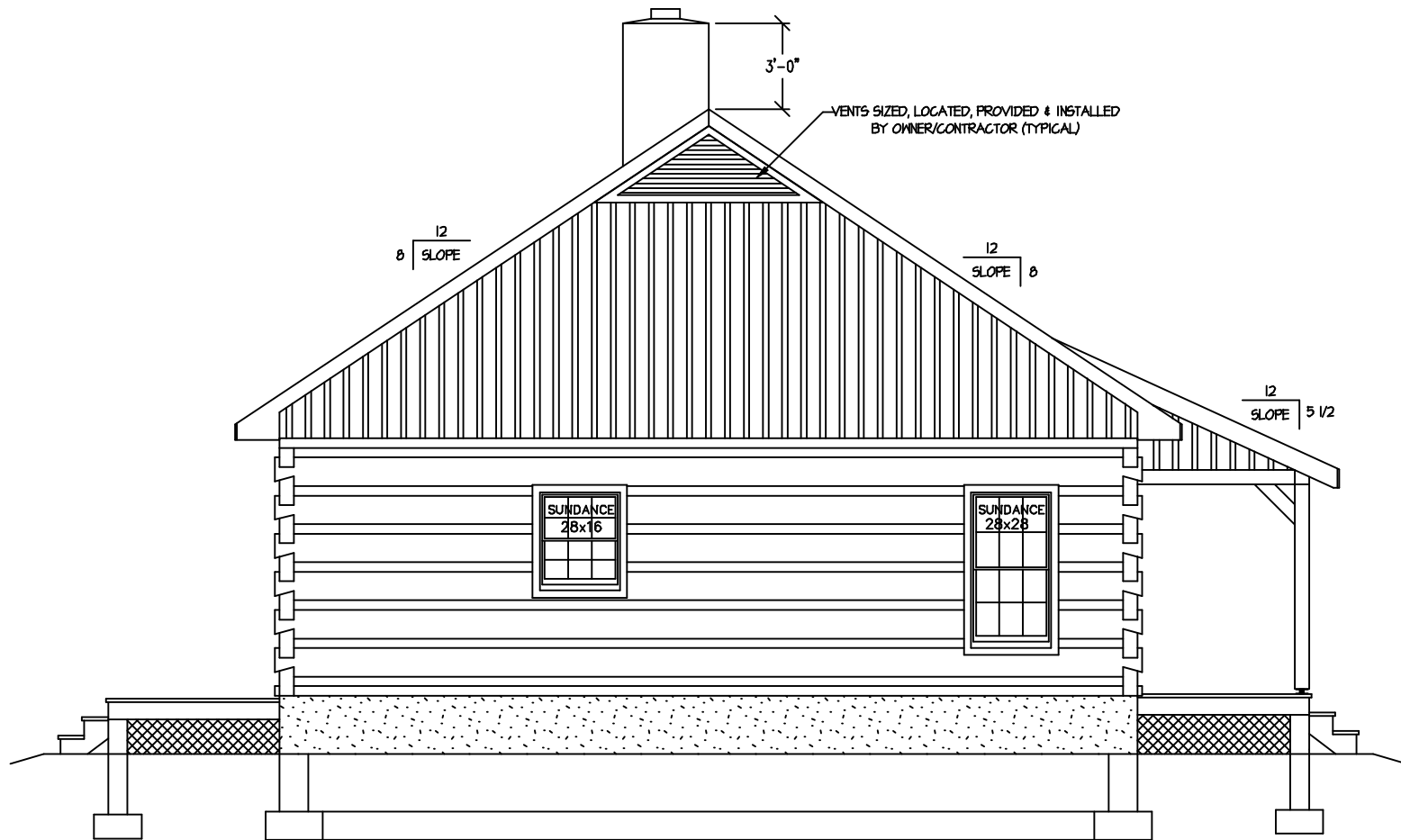
PLAN LEFT
