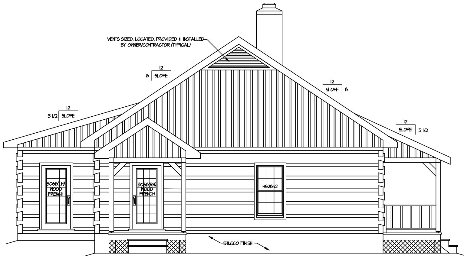
PLAN LEFT
