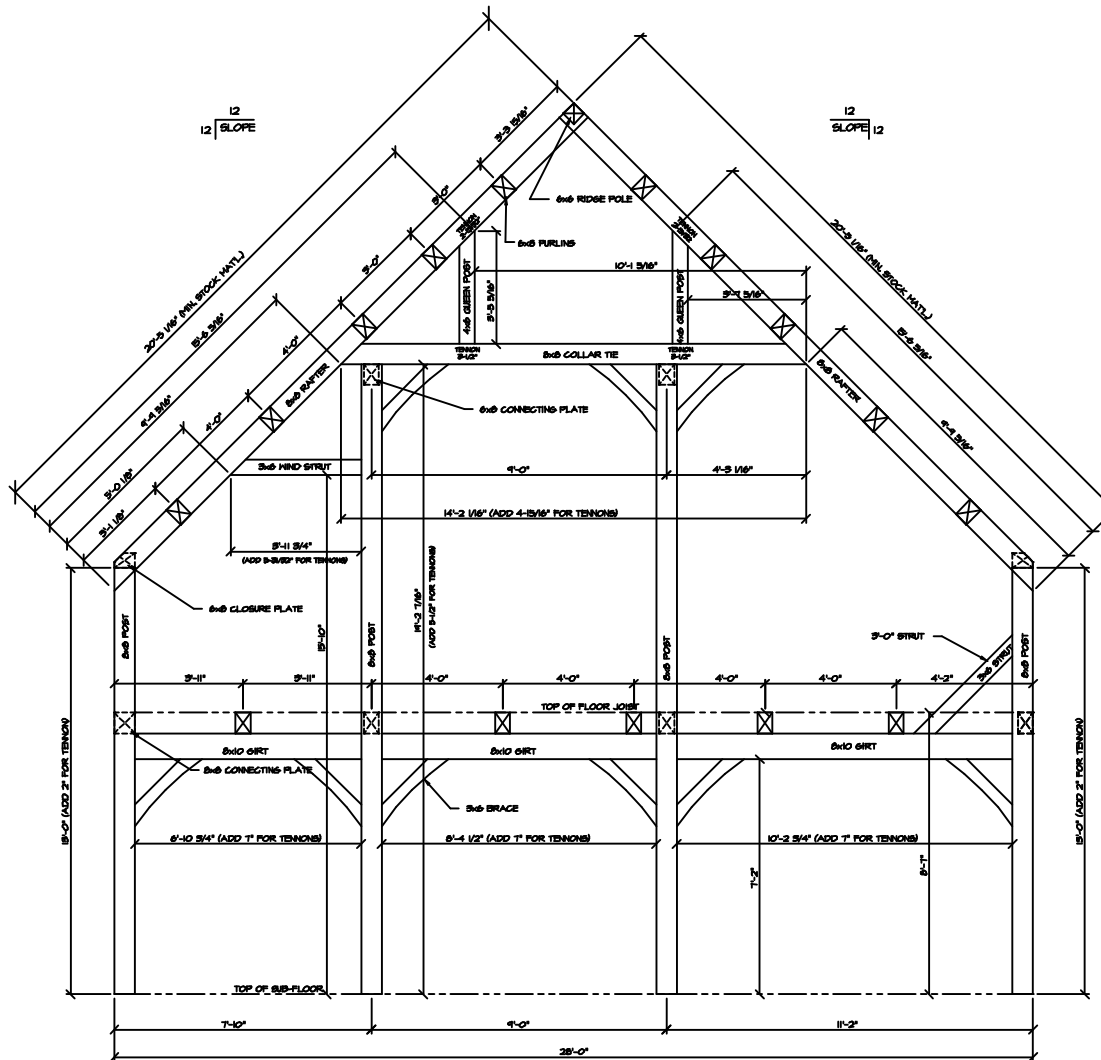
BENT 2
