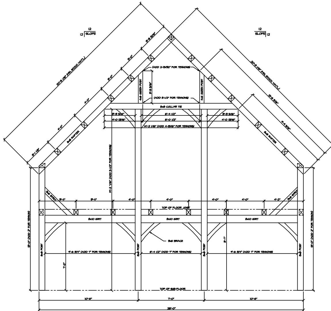
BENT 1
