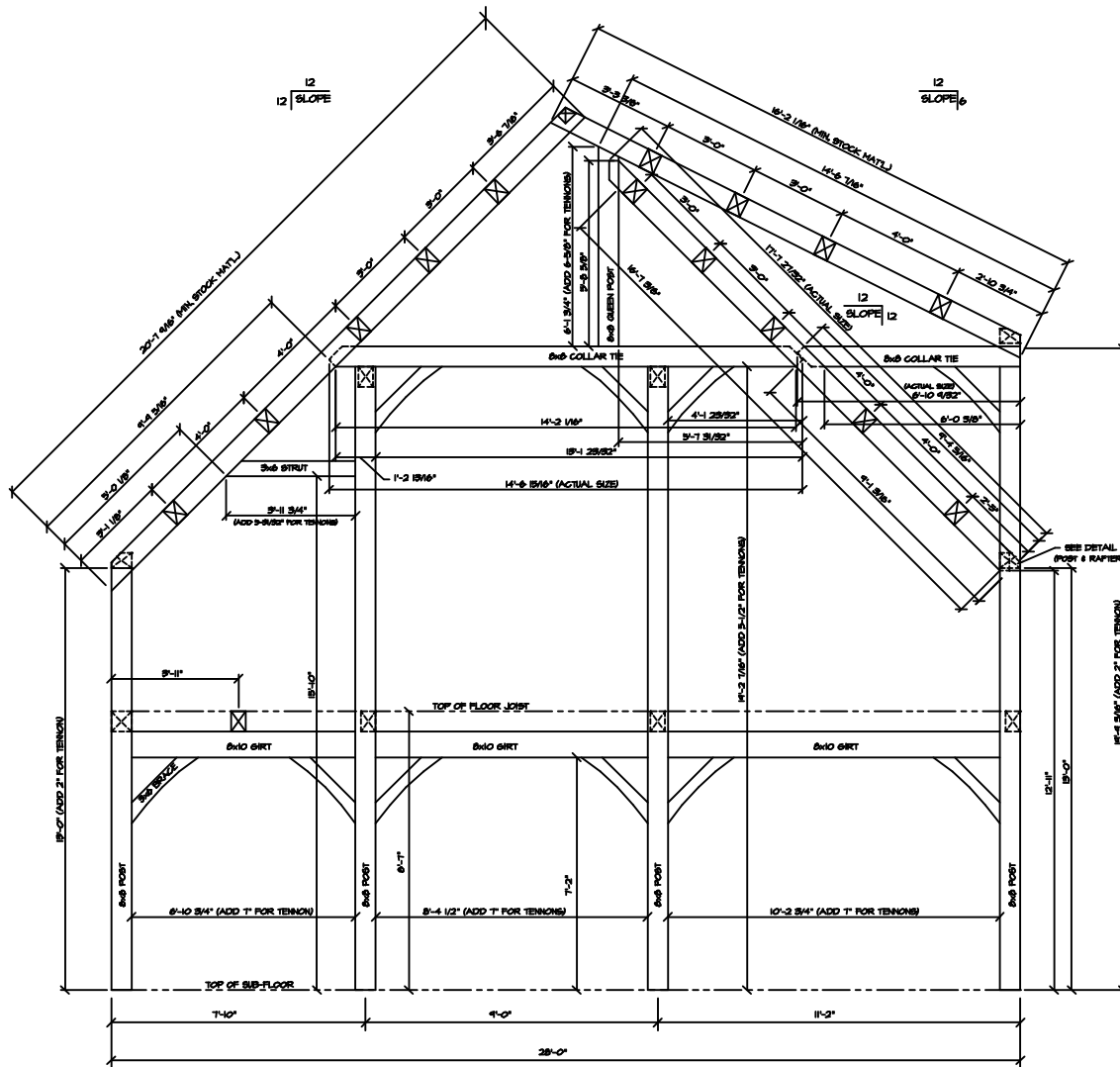
BENT 3 SCALE: 1/2" = 1'-0"
