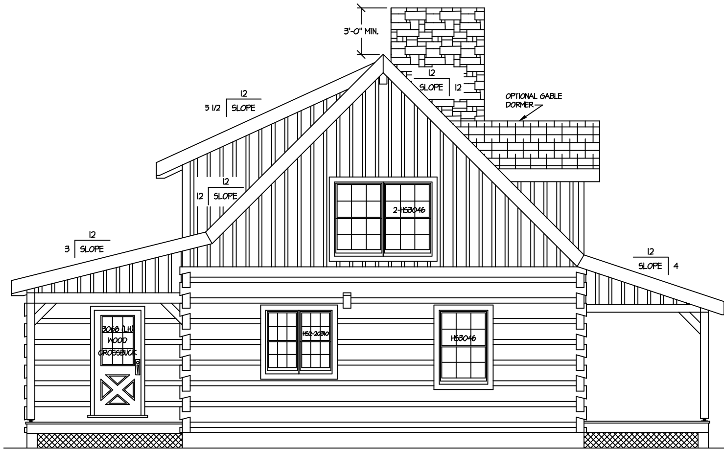
PLAN LEFT
