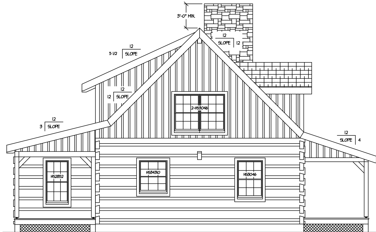
PLAN LEFT
