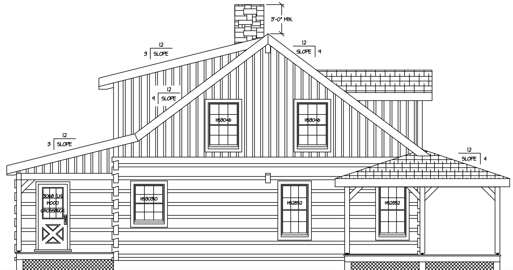
PLAN LEFT
