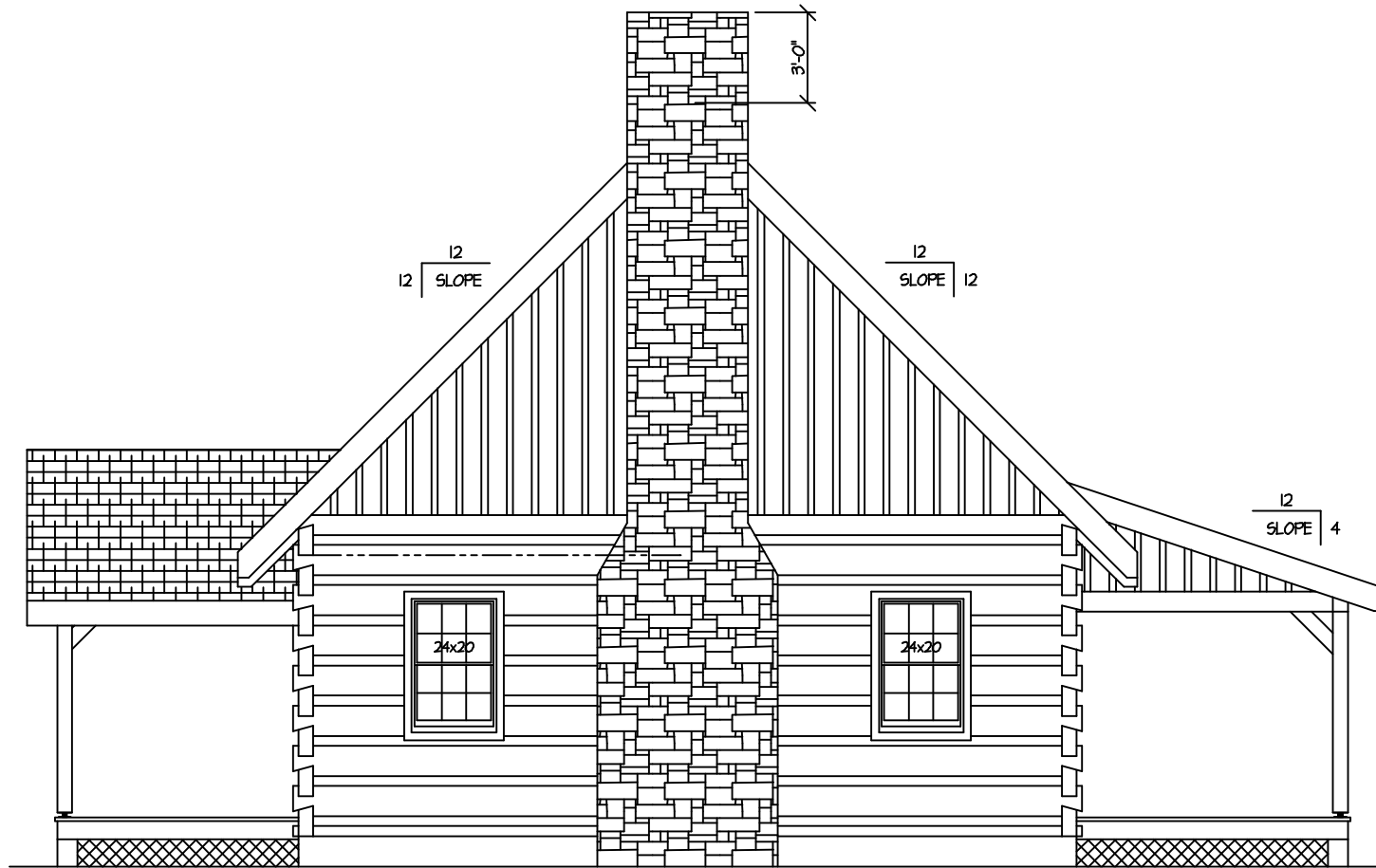
PLAN LEFT
